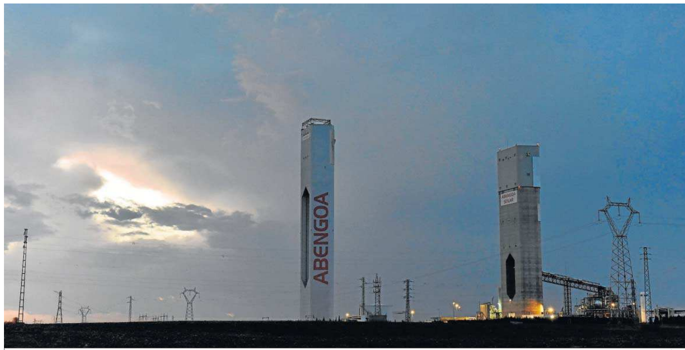
Planta termosolar construida por Abengoa en Santlúcar la Mayor, en Sevilla.
