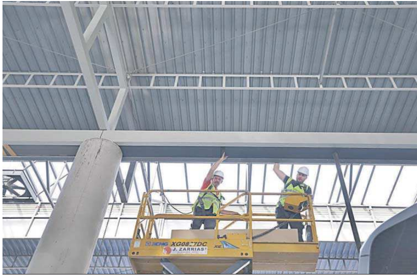
Los falsos techos se han desmontado casi por completo en los 10.000 m2 de andenes y dársenas.
